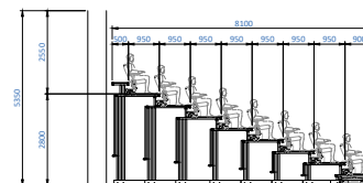
Sección SC 1/100
