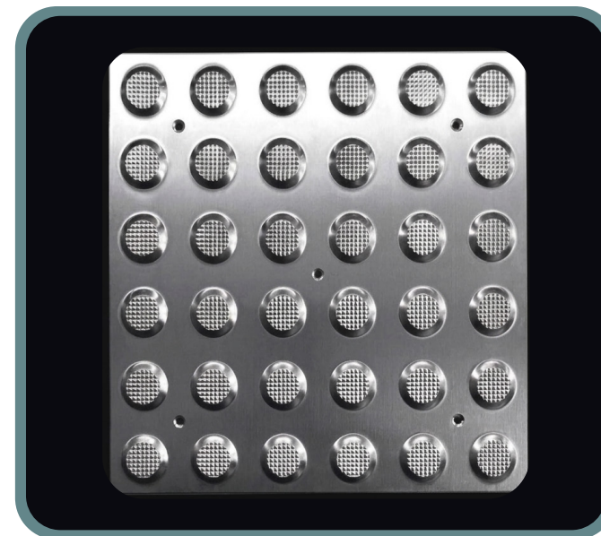
Patrón ondulado puntual antideslizante fresado
