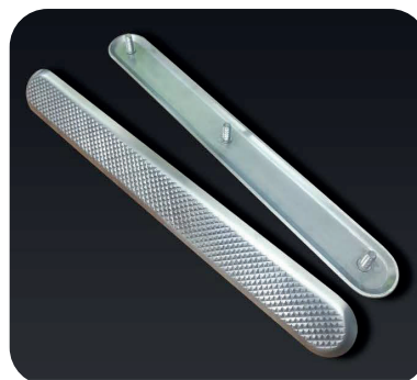
Banda podotáctil con patrón ondulado antideslizante fresado
