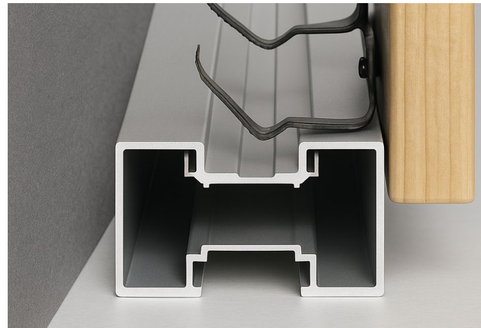
Revestimiento con Madera 15 mm
